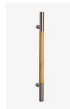
VP-19D Ø30 mm, einseitig, Edelstahl, matt/Holz, Stützen gerade /
